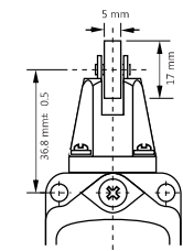
Top Roller Plunger
