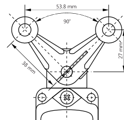
Yoke Roller Lever
