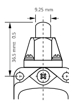
Top Plunger
